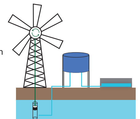
Schéma : prélèvement dans un cours d'eau par pompage éolien
